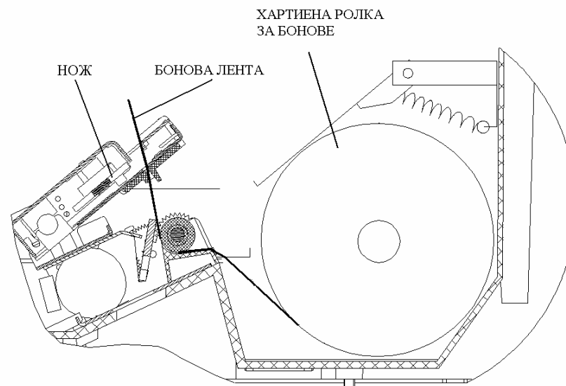
Фиг. 4 Поставяне на бонова лента
