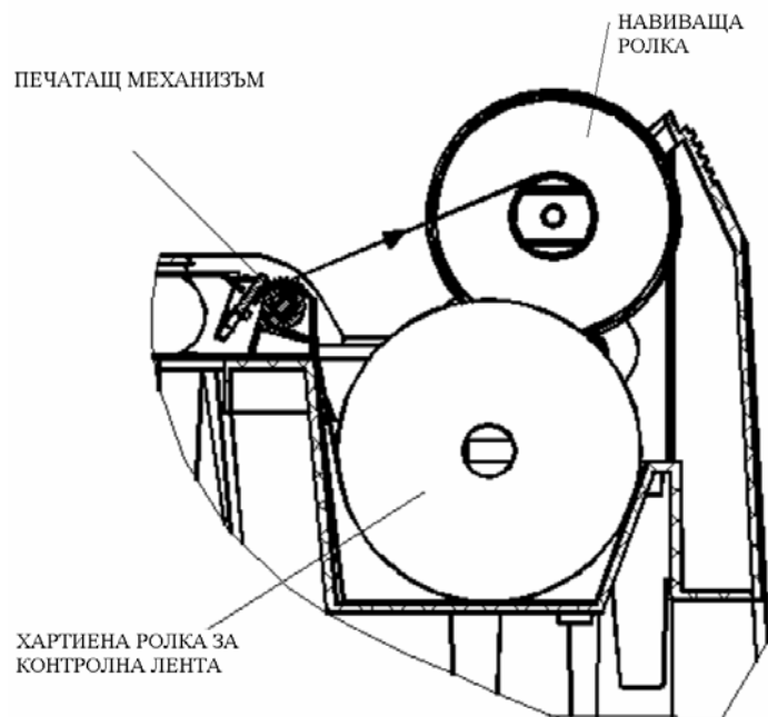
Фиг.5 Поставяне на контролна лента
