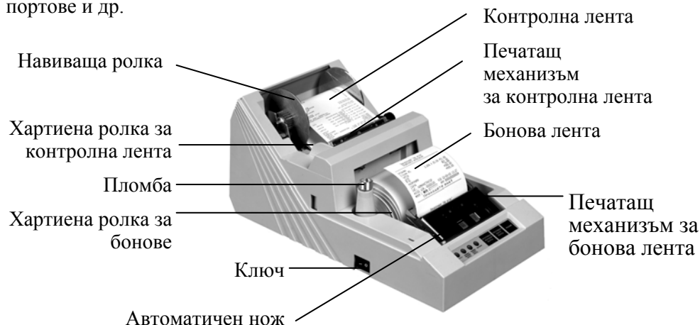
Фиг.1 Вид на фискалния принтер без капак
